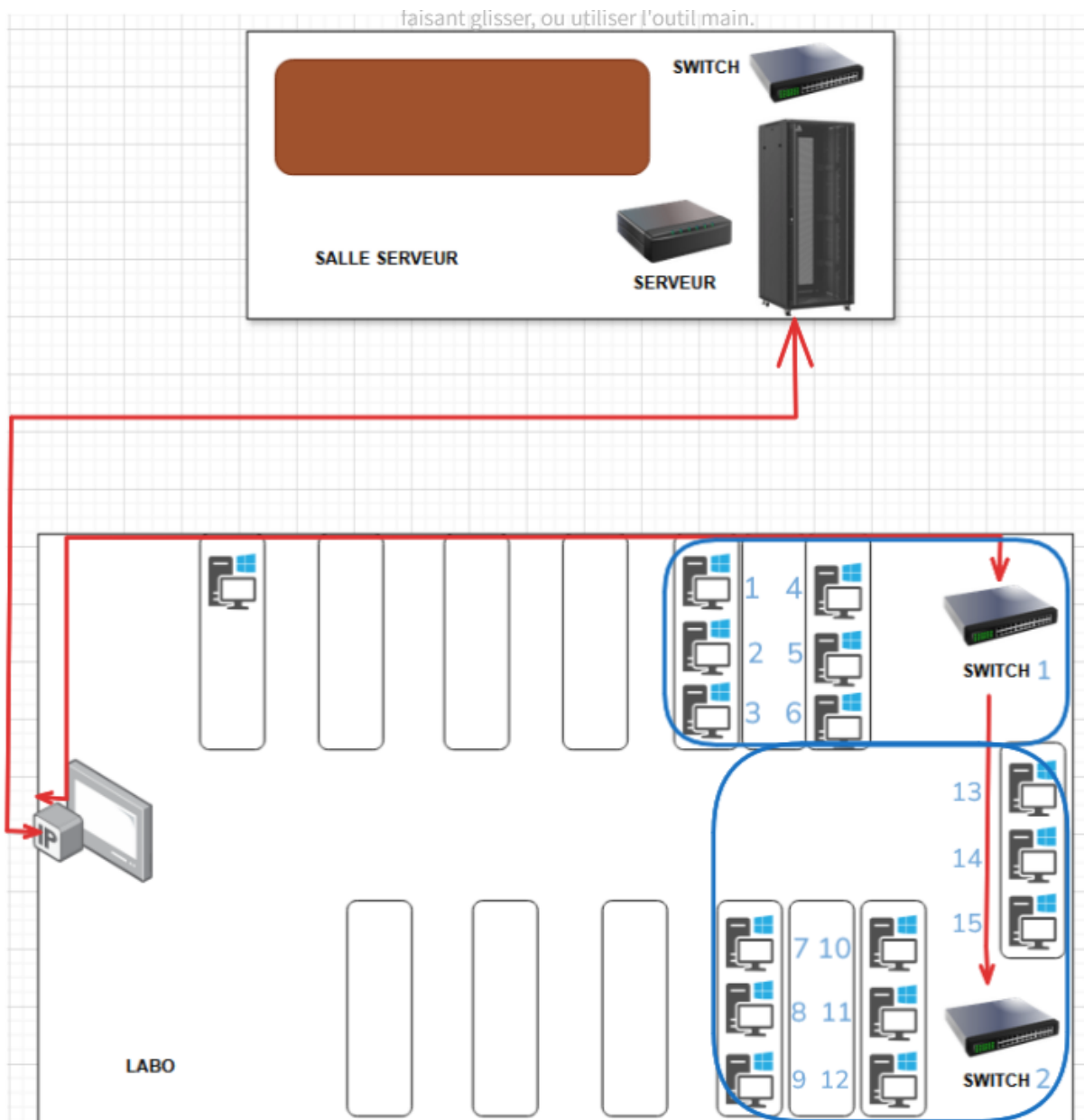
Schéma infrastructure réseau entre salle serveur et labo
